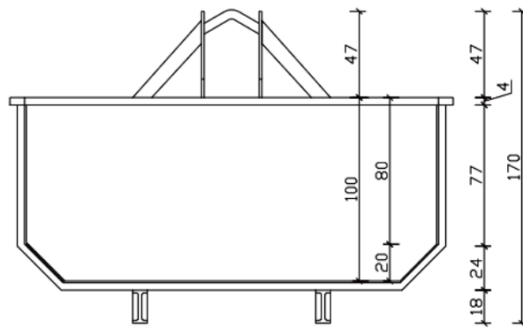
COUPE PARTIELLE B-B
